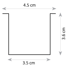
פרופיל 35/35 שקוע
