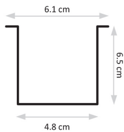
פרופיל 50/70 שקוע
