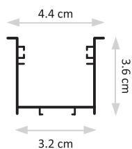
פרופיל אולטרא שקוע
