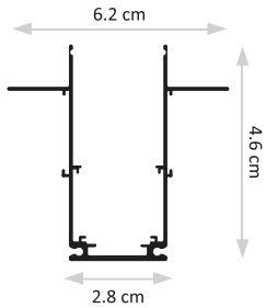
פרופיל מגנט טרימלס שקוע
