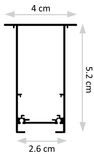
פרופיל מגנט שקוע
