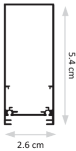
פרופיל מגנט
