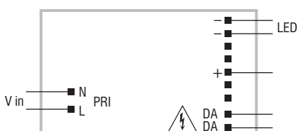
Collegamento DALI
